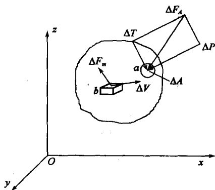
图 1-1 表面力和质量力
