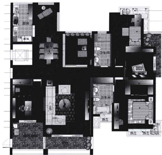
平面布置图
