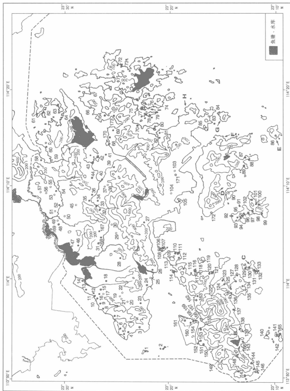
● 史学时代遗址 ○ 史前及历史时代遗址 ← 历史时代遗址 ▲ 史前时代石刻 ■ 明代沉船遗址 图一 香港考古遗址及古石刻分布示意图(遗址及古石刻名称见附录)
