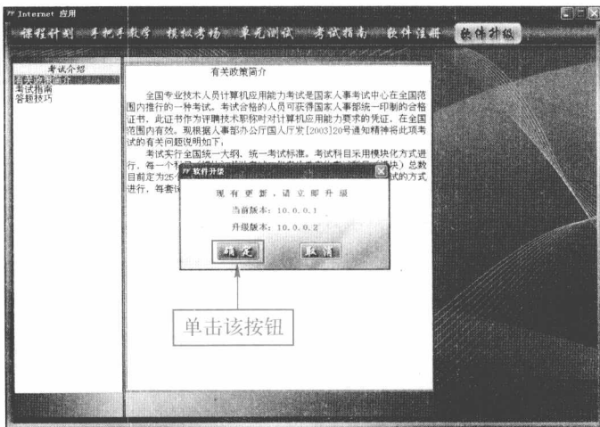
图 19 升级提示
