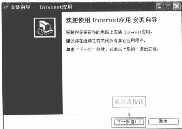
图 2 欢迎界面
