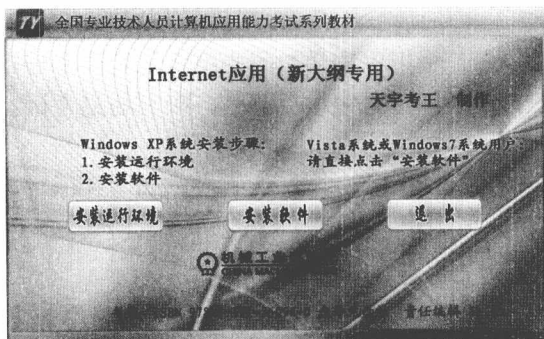
图 1 主界面
