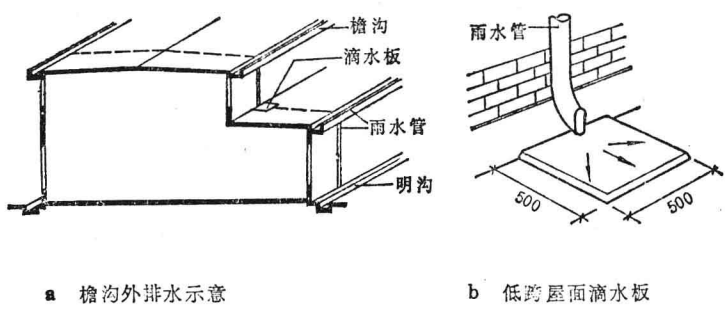
图 8-7 高低跨处设滴水板
