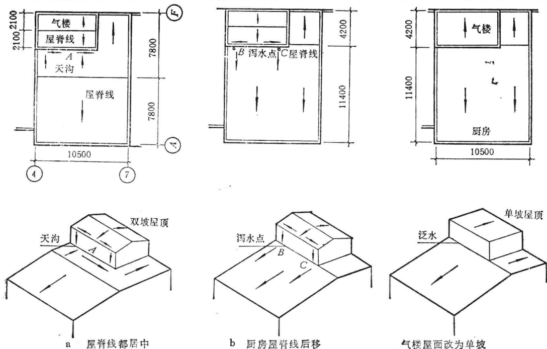
图 8-6 某厨房屋面排水组织分析
