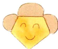
氧化铝
