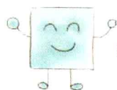
氯化钠
