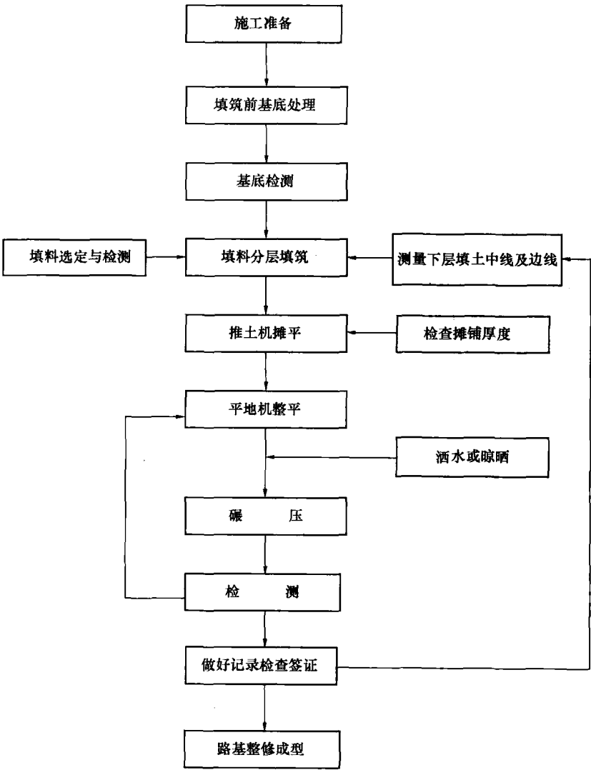
图 2B311014 土方路堤填筑施工工艺流程图
