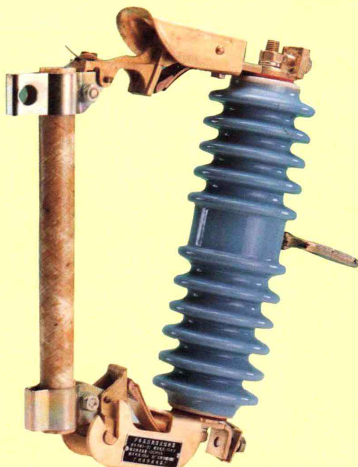
10KV戶外交流高壓跌落式熔斷器
