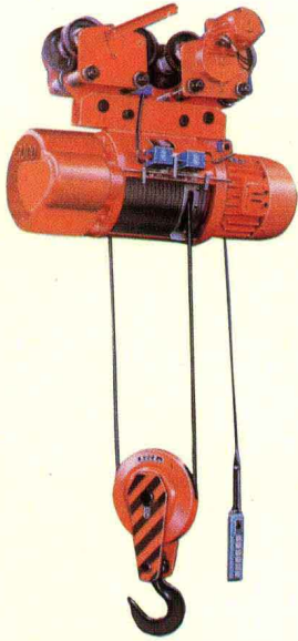
CDI型電動葫蘆 起重量：0.5-5噸
