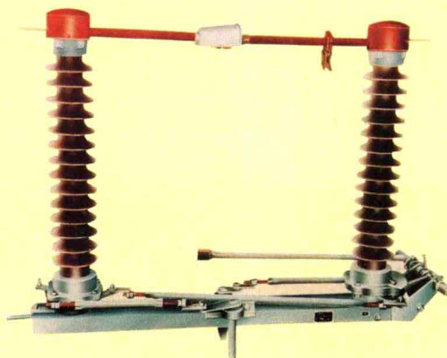
10、35、110KV戶內、戶外高壓隔離開關
