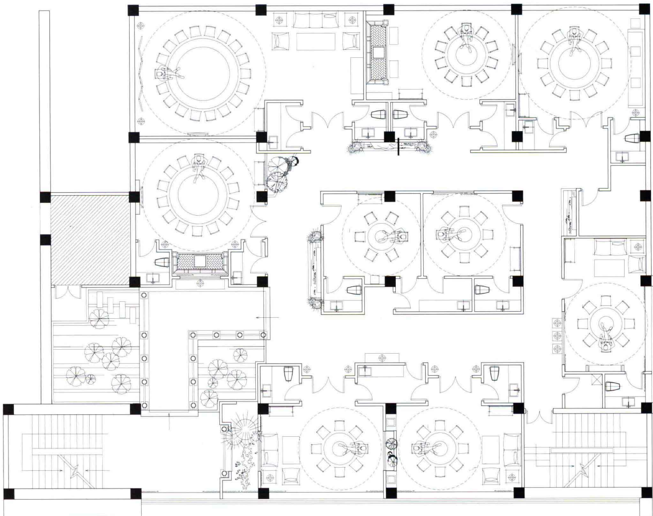
三层平面布置图
