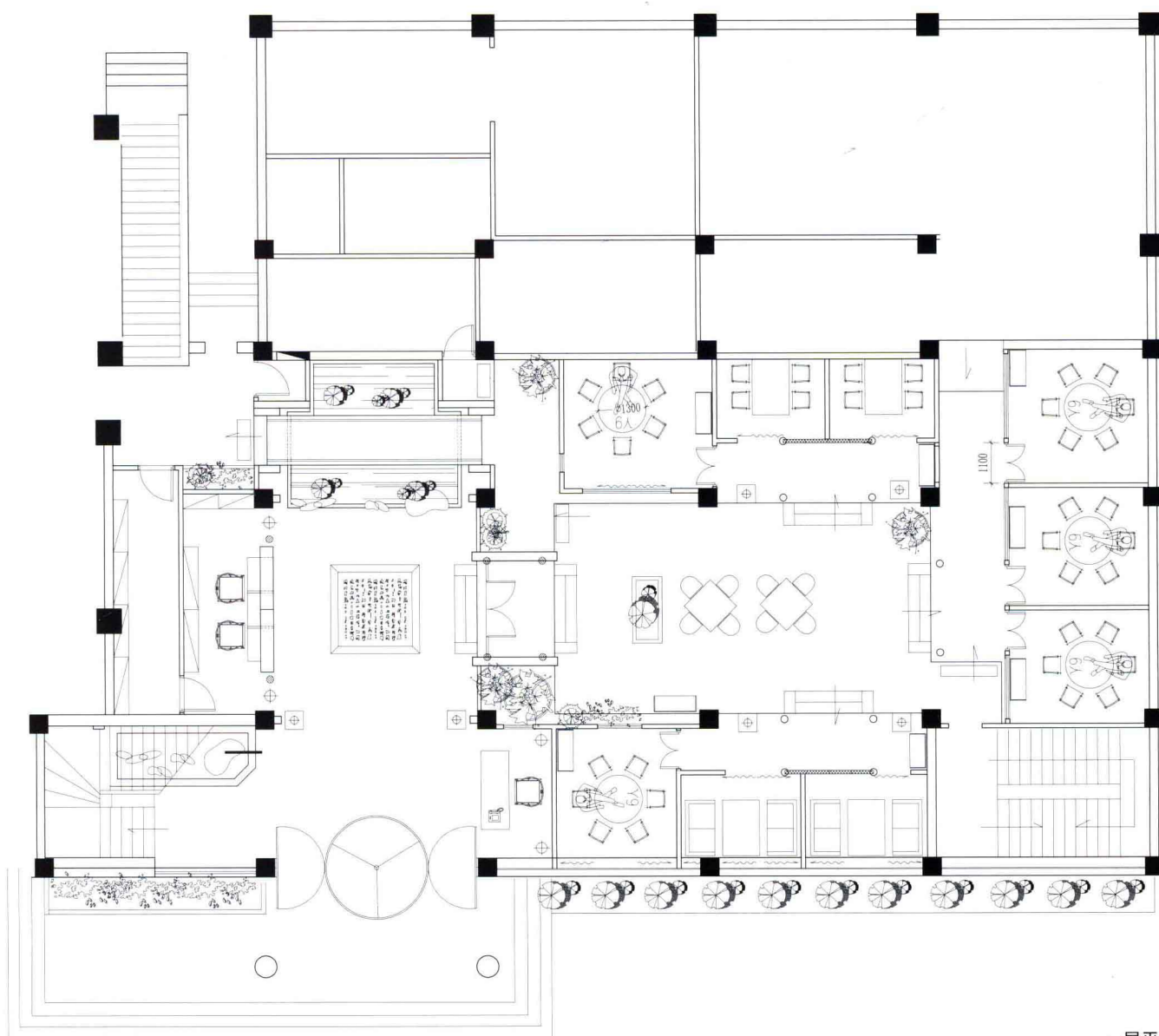
一层平面布置图
