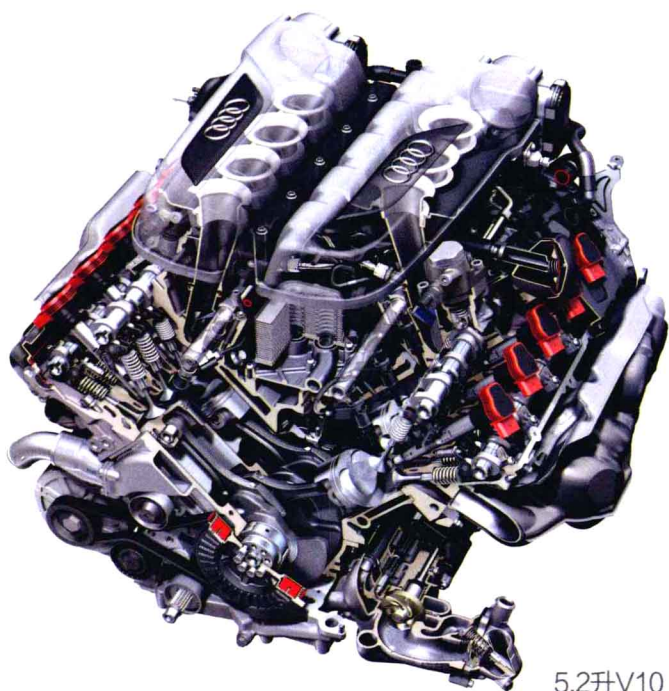
5.2升V10 FSI发动机
