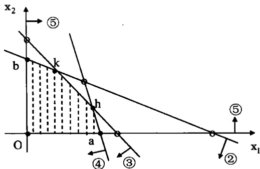
图 1-1 数学模型的可行解域
