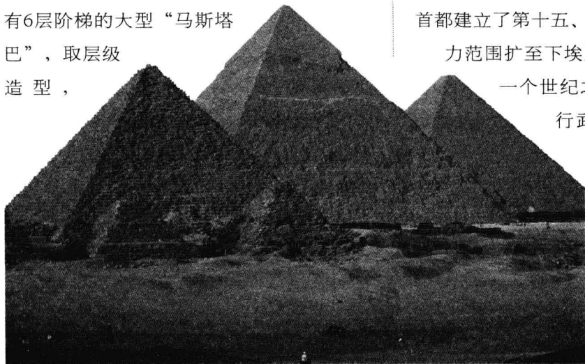
◆ 胡夫金字塔
