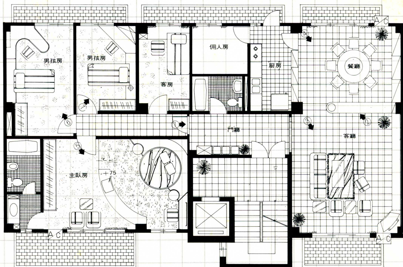
平面圖 1:100cm
