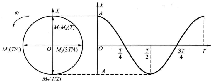
图 11-7 旋转矢量图和简谐振动的 x-t 图
