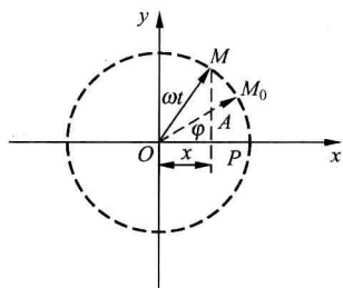
图 11-6 旋转矢量图
