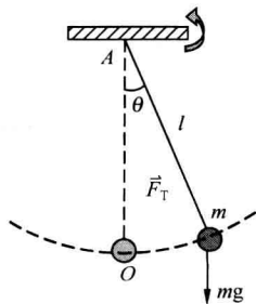
图 11-13 单摆
