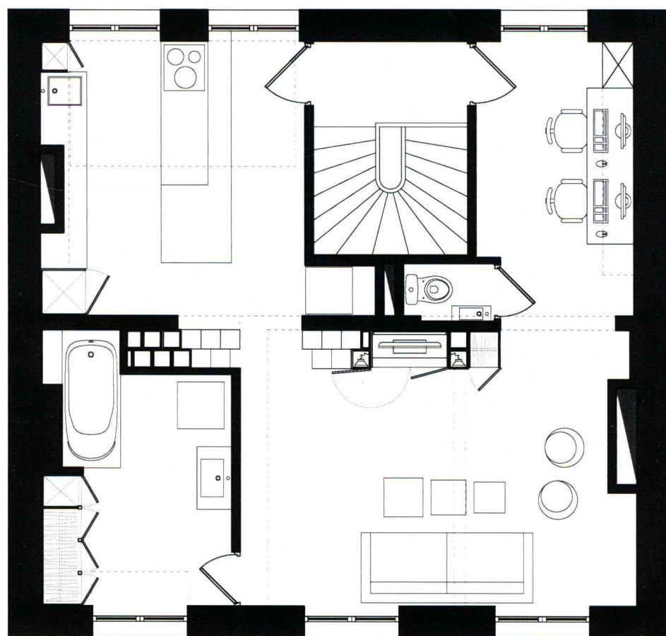
底楼平面图
