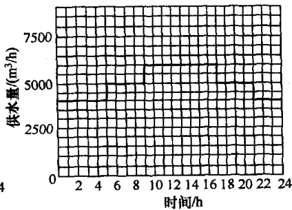
图2 二级泵房供水量变化曲线
