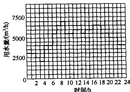
图1 用水量变化曲线
