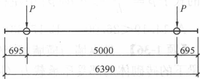
图 1-29-1 吊车轮压及轮距
