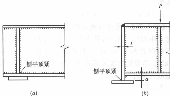
图 1-20-1 梁的支承加劲肋 (a) 平板支座；(b) 突缘支座
