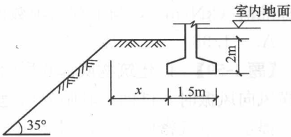
图 1-54-1 基础位置
