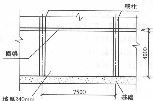
图 1-43-1 外墙立面
