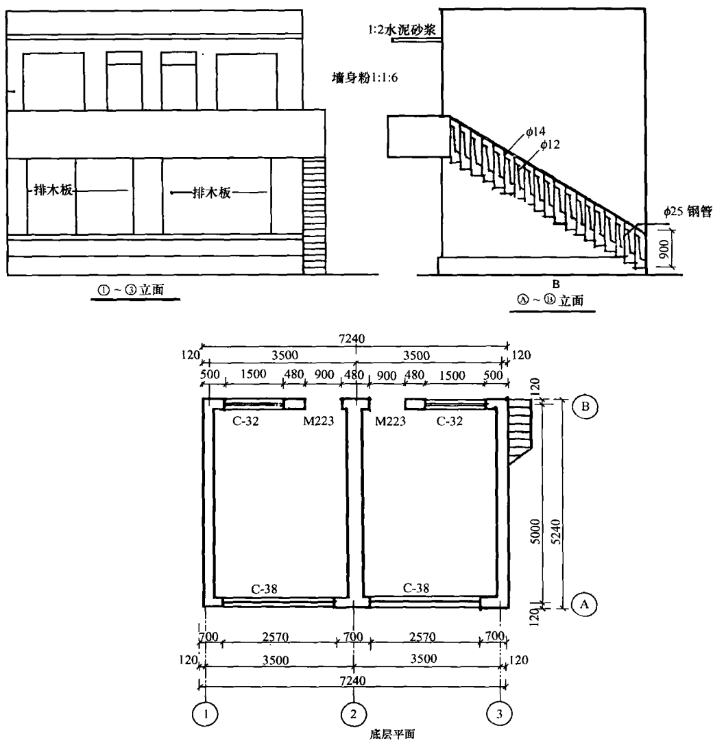
图 1-1-1 某小百货楼工程底层平面及立面图
