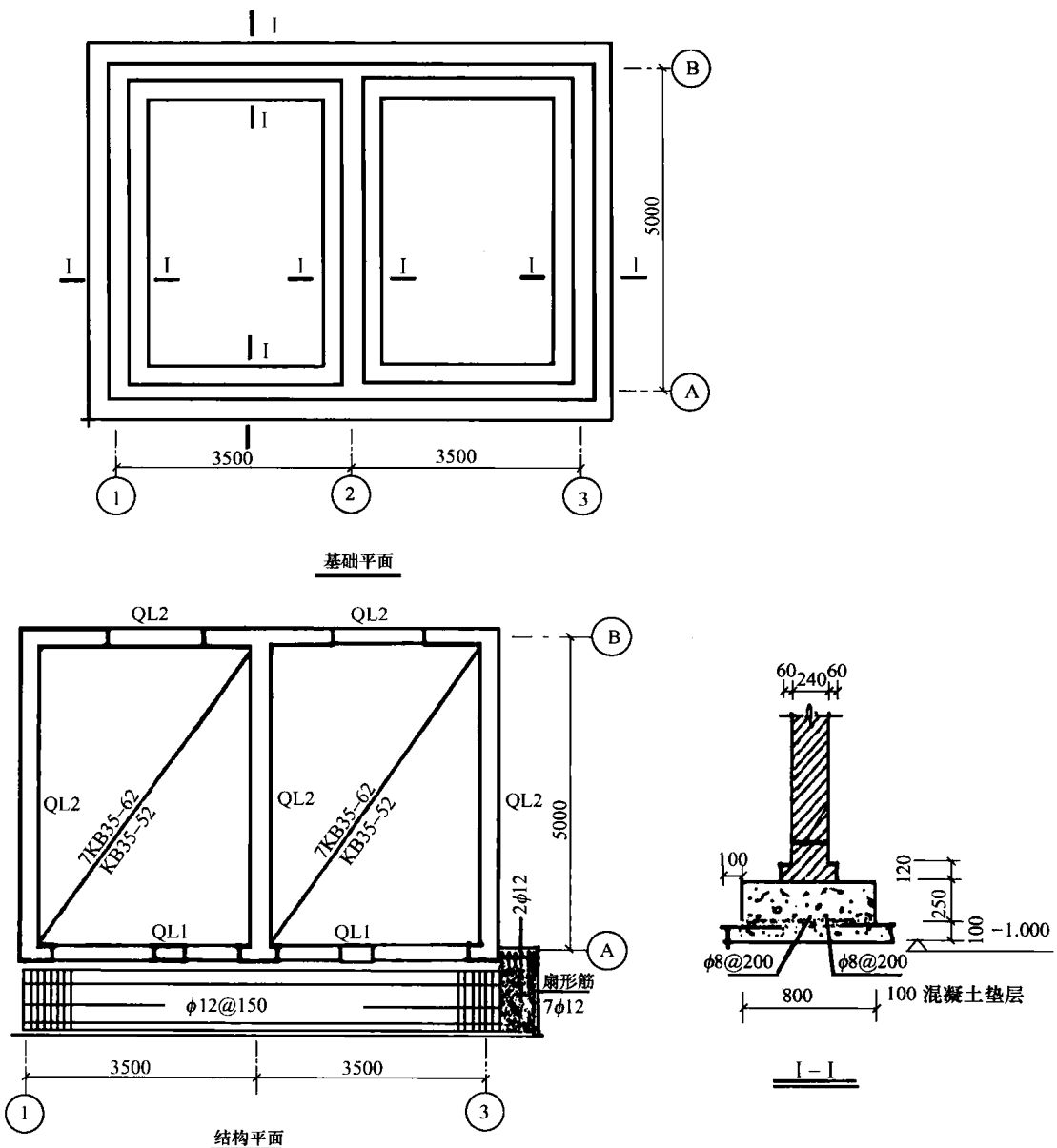
图 1-1-3 某小百货楼工程基础结构图
