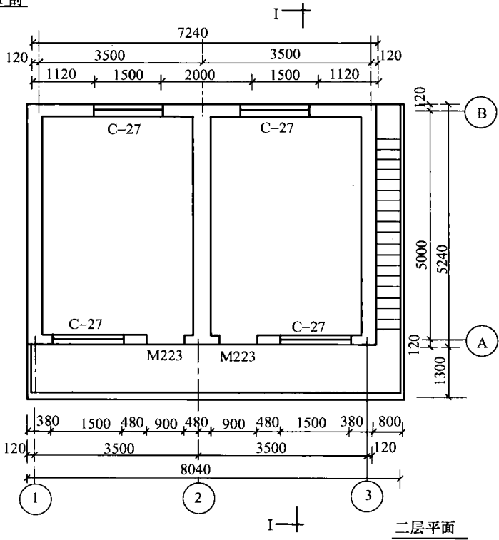
图 1-1-2 某小百货楼工程二层平面及剖面图
