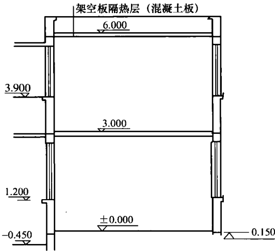
I—I 剖
