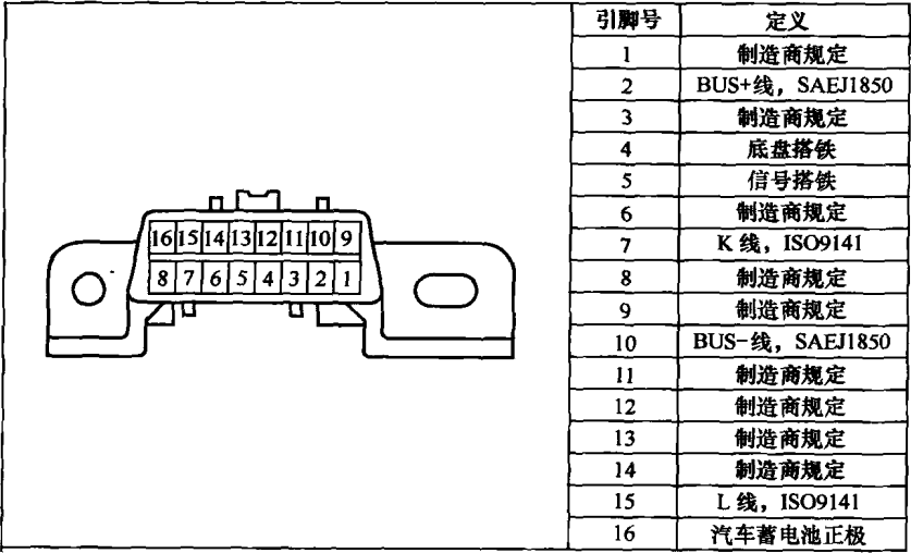
图 1-1 OBD II 故障诊断连接器
