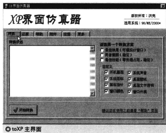
toXP 主界面
