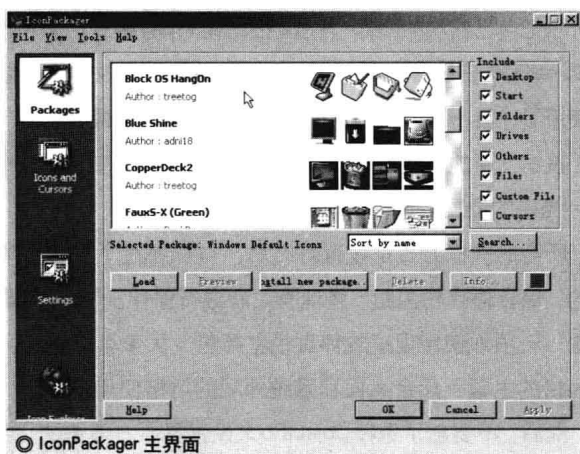
IconPackager 主界面
