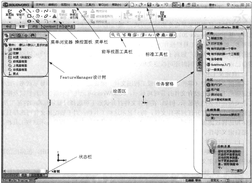
图1-1 Solidworks 2012界面
