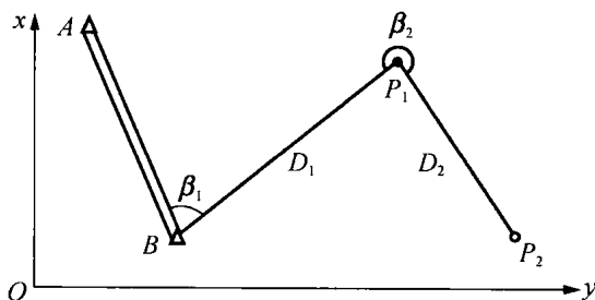
图 0-8 地面点平面位置的确定
