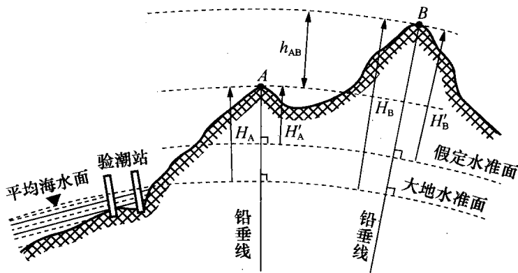
图 0-6 高程与高差的定义及其相互关系
