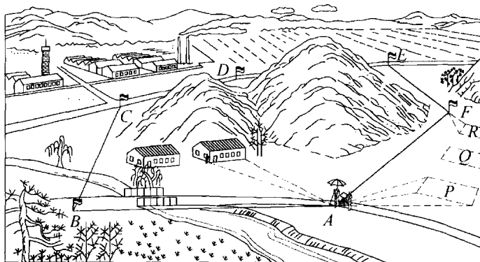
图 0-10 地物和地貌
