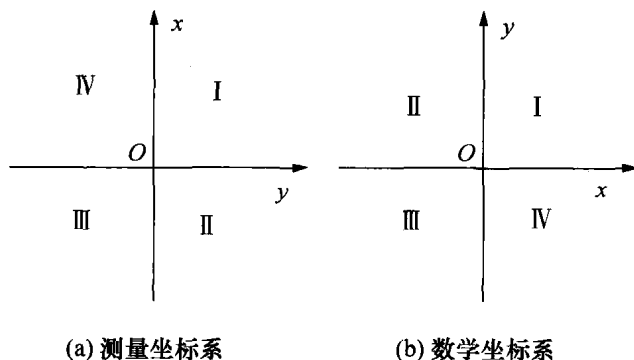
图 0-3 测量坐标系和数学坐标系
