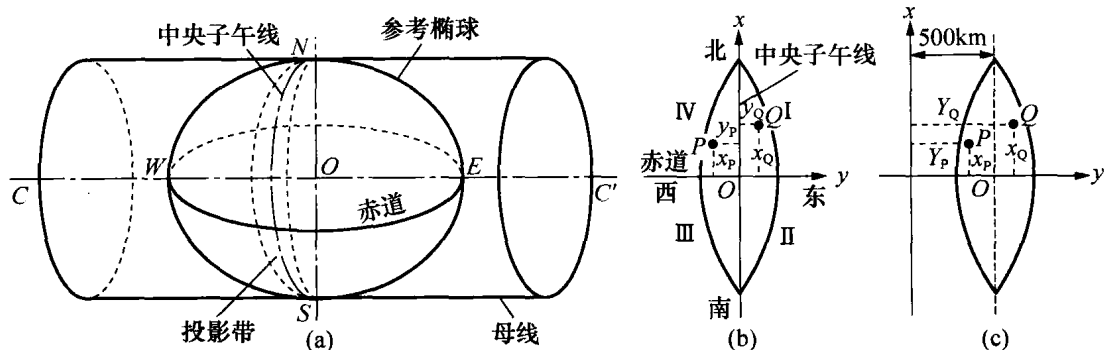
图 0-4 高斯平面坐标系投影图
