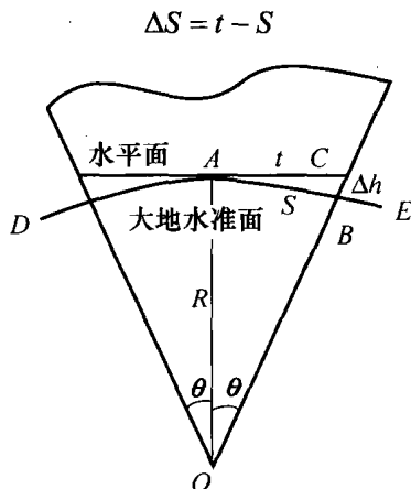
图 0-7 地球曲率对水平距离的影响
