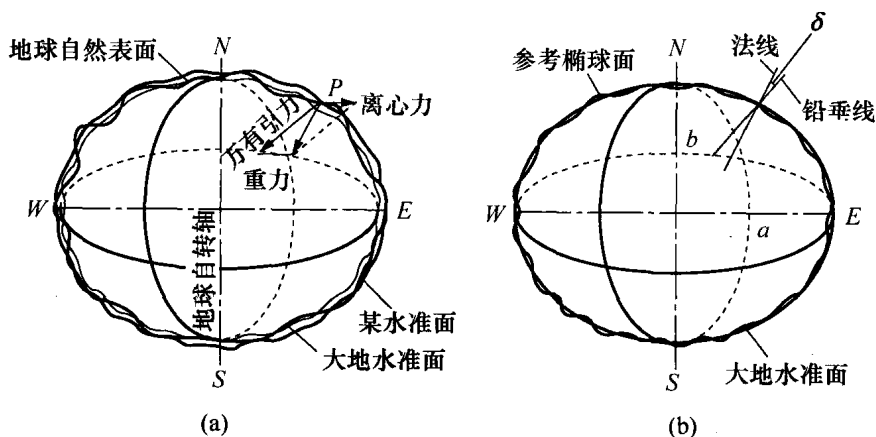
图 0-2 地球自然表面、水准面、大地水准面、参考椭球面、铅垂线、法线间的关系
