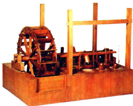
连击水碓 西汉
