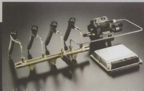
共轨系统
