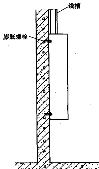
图 1-11 壁挂式配线箱的安装
