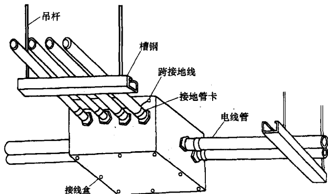
图 1-5 室内接线盒做法
