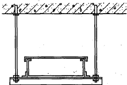
图 1-6 线槽水平安装方法
