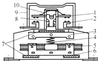
图 1-3 接触器的外形及结构
