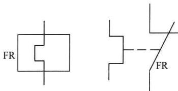
(a) 热继电器的驱动元件 (b) 动断触点
