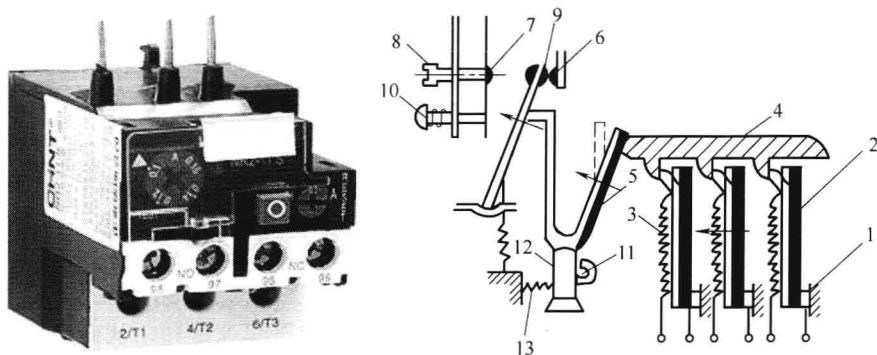
图 1-7 热继电器外形及结构
