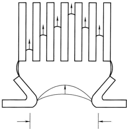
图 1-4 接触器主触点的电弧
