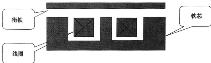
图 1-1 电磁机构
