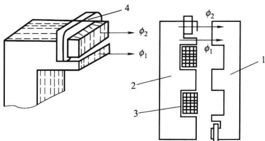
图 1-5 交流接触器的短路环
