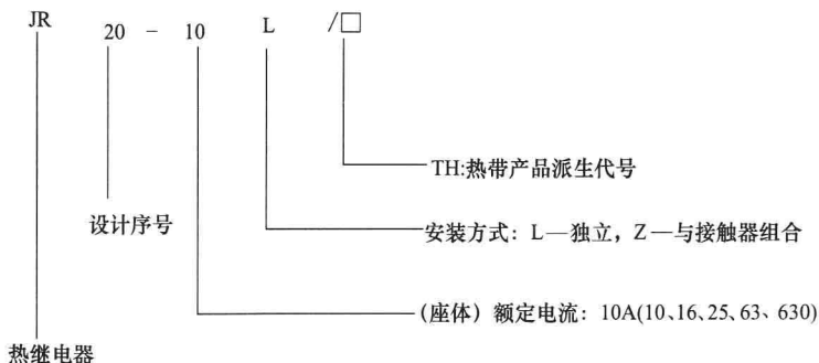
图 1-9 热继电器的型号规格
