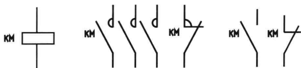
图 1-6 接触器的符号表示
