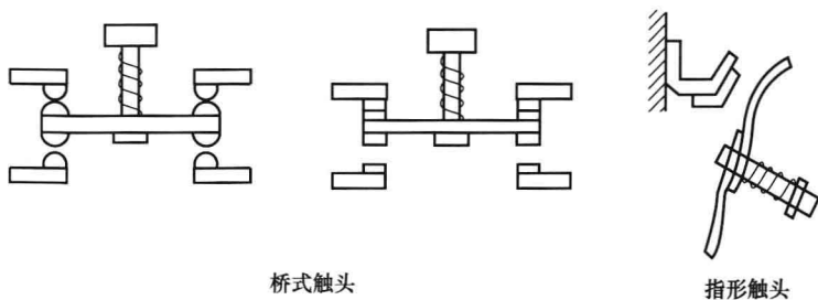
图 1-2 触头的结构形式
