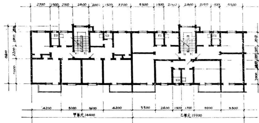
平面 1:150
