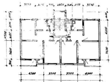
甲单元平面
