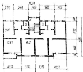
甲单元平面
