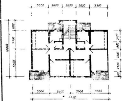
甲单元平面 1:200
