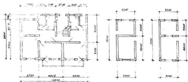
甲單元平面
