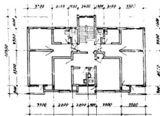
乙单元平面
