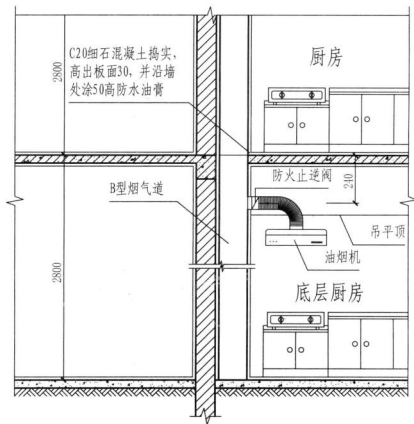
B型烟气道安装示意图
