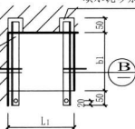
楼板承托平面一
