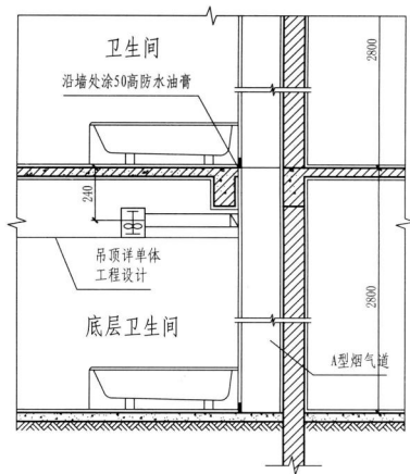
A型烟气道安装示意图
