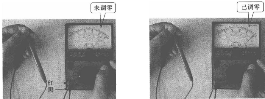
图 1-6 指针型万用表表针调“0”示意图
