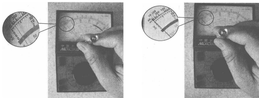
图 1-4 指针型万用表表针复位的调整
