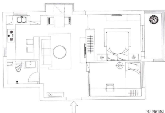
平面图
