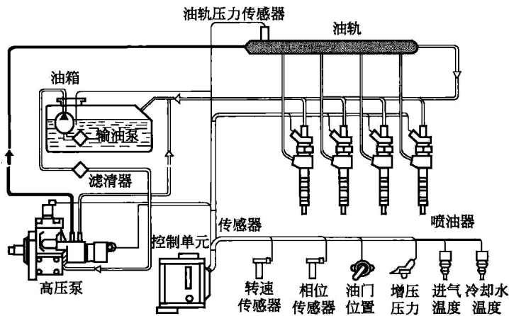
图 1-6 高压共轨系统组成图
