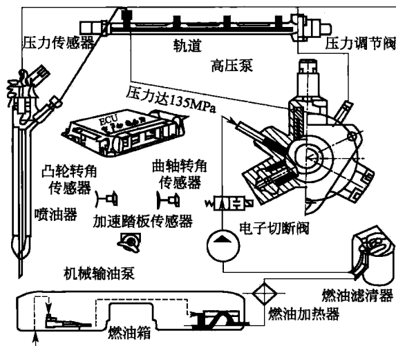
图 1-5 UNIJET 型电控共轨燃油系统
