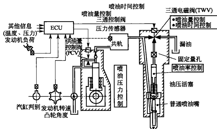
图 1-4 ECD-U2 共轨系统（早期）
