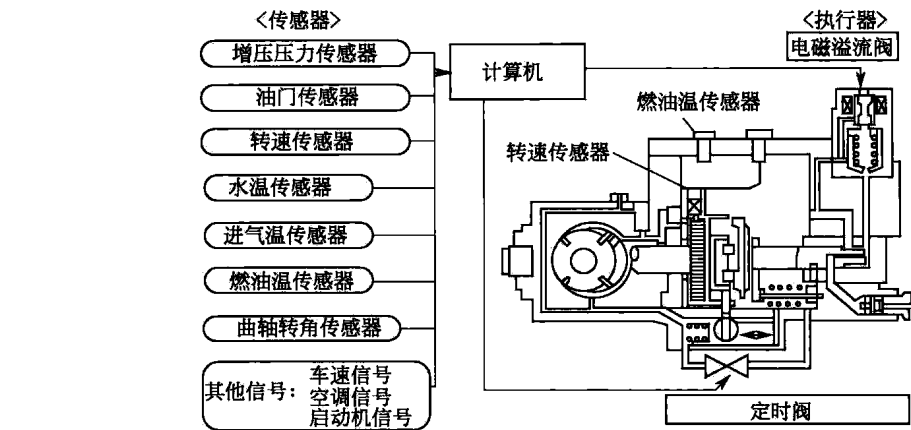
图 1-1 典型的电控分配泵的系统图
