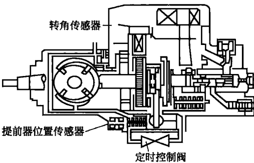
图 1-2 电控分配泵——位置控制式
