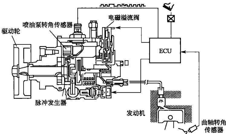
图 1-3 时间控制式电控分配泵系统
