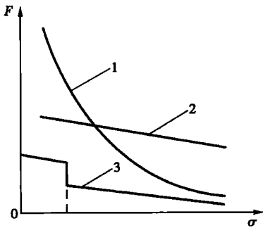
图 1.2 电磁铁的吸力特性曲线
