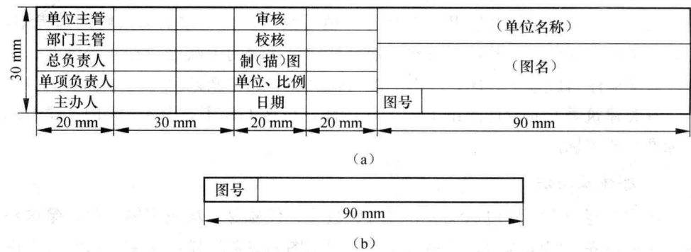
图 1-2 通信工程勘察设计常用图街
