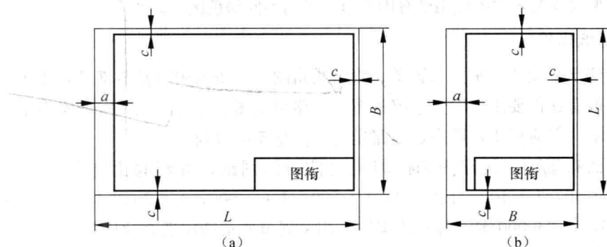
图 1-1 图框格式
