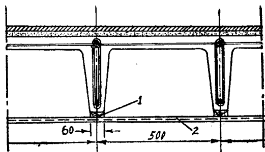
圖 1 一體式多肋樓板
