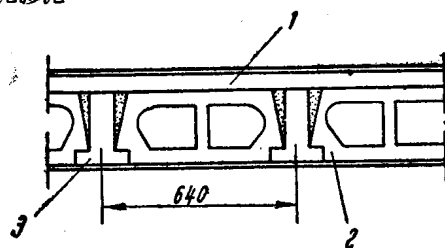
圖 2 純裝配式多肋樓板
