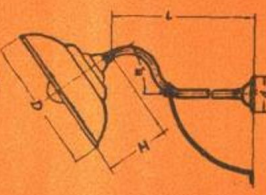
GC3-F30°弯杆灯
