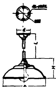
GC3-A直杆吊灯
