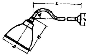
GC5-D 90°弯杆灯 GC5-E 60°弯杆灯
