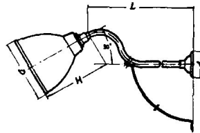
GC5-F 30°弯杆灯
