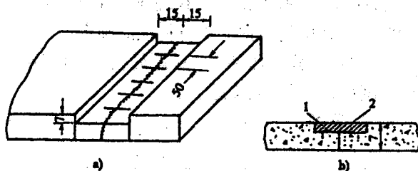
图 7.1.2 条带补缝(单位:cm)
