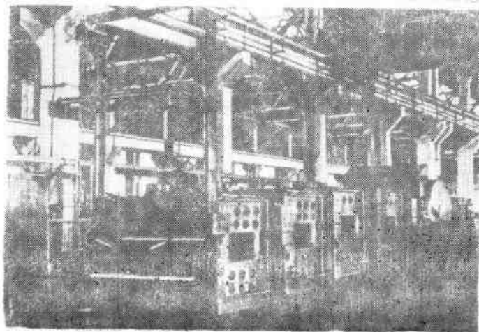
CGLMA045型轧卷式平幅练漂联合机，适用于纯棉，与棉化纤混纺织物烧毛后煮练漂白之用。
