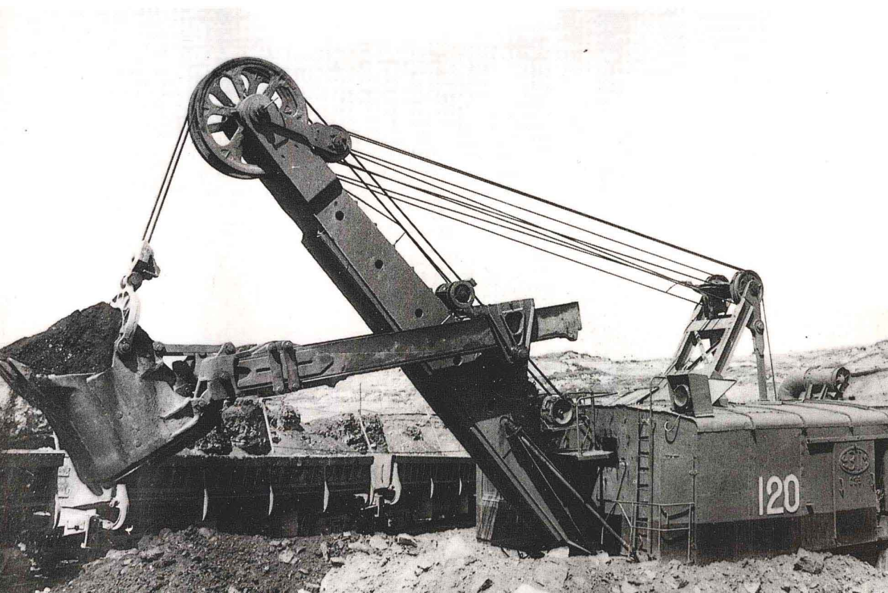
▼露天矿电镐作业现场
