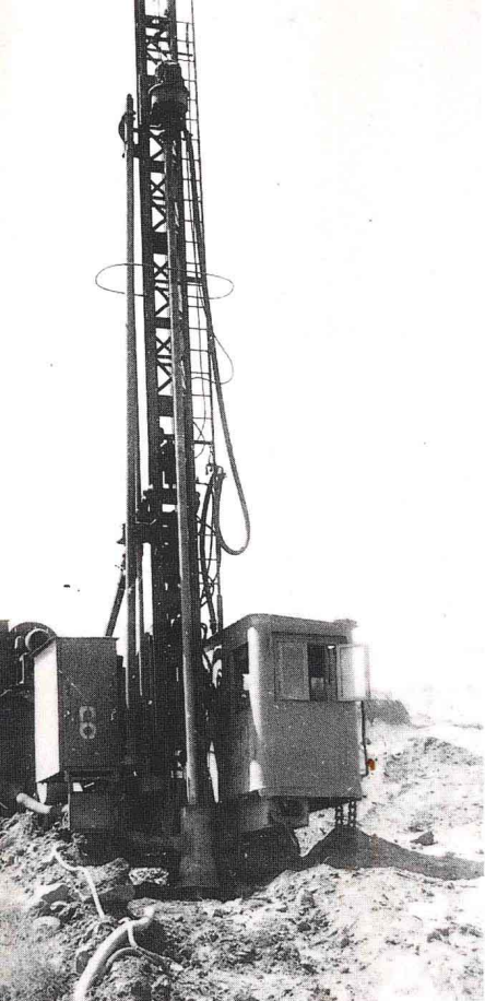
▲露天矿潜孔钻
