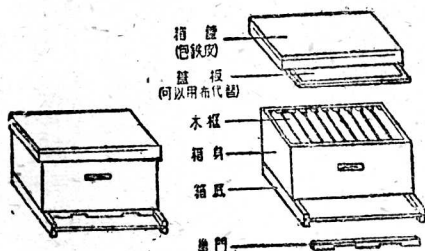
图1 十框式蜂箱
