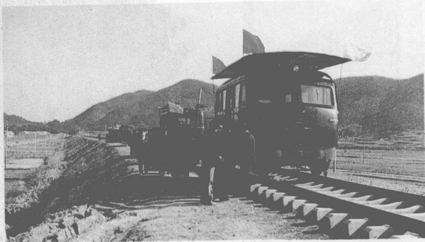
北仑铁路鄞县段正在接轨。
