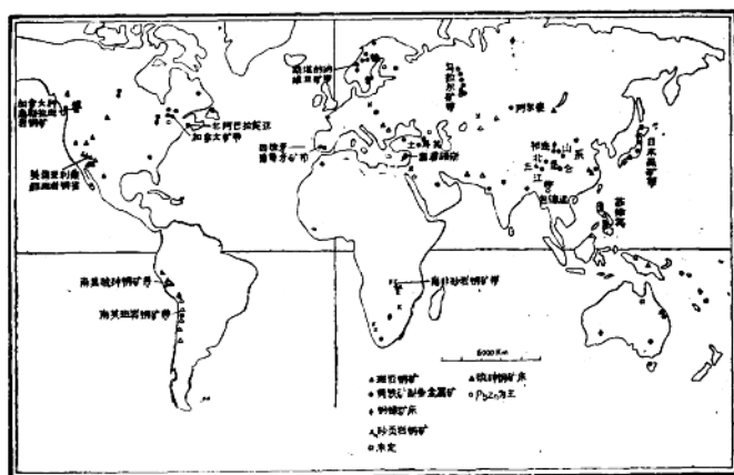
图1 世界火山成因铜、铅、锌和其它类型矿分布简图 (根据狄克逊矿床分布图16加以补充合并及简化)
