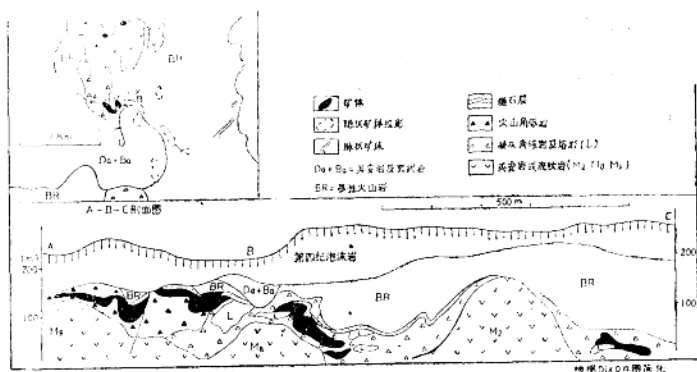
图2 日本Kosaka区黑矿矿体示意图 (根据Dixon图简化)
