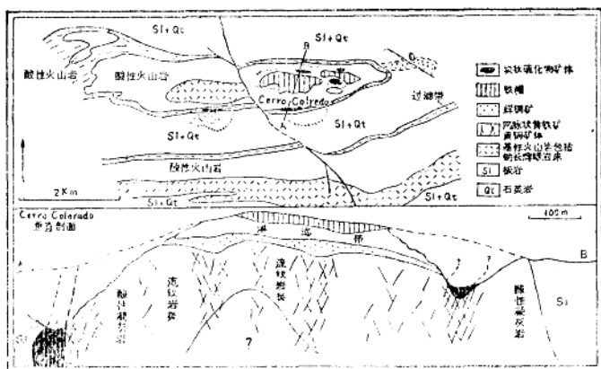
图3 西班牙里奥奥托矿区地质简图 (根据Dison图简化)
