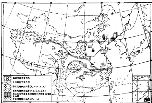
图5 中国太古界一下元古界和各地质时期火山岩分布示意图 （根据中华人民共和国地质图集和一些1:20万地质图编制）
