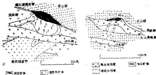
图4 加拿大一些与酸性火山岩有关的矿床 (根据Sangster简化)
