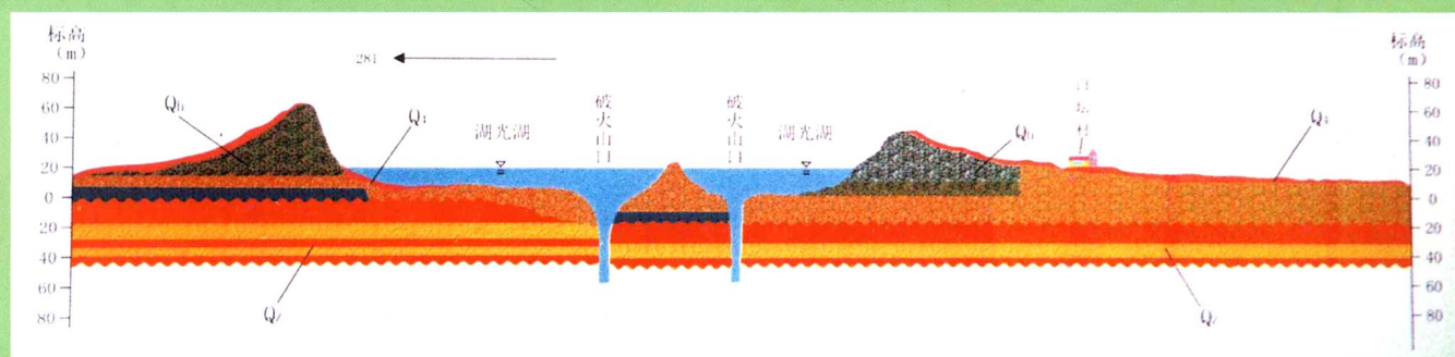
湖光岩地质剖面图
