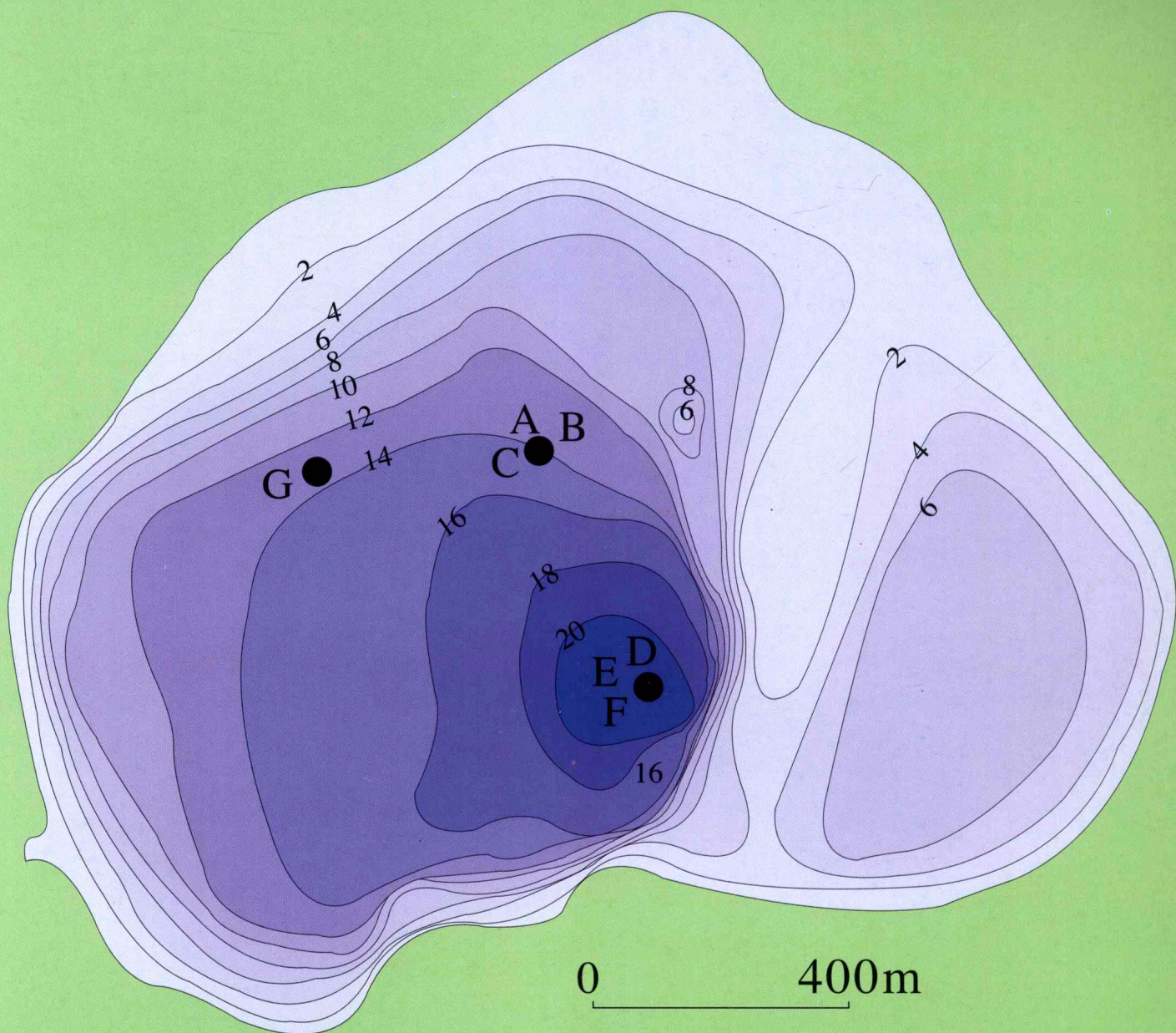
湖光岩湖水等深线图
