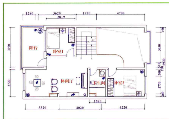
三层平面图
