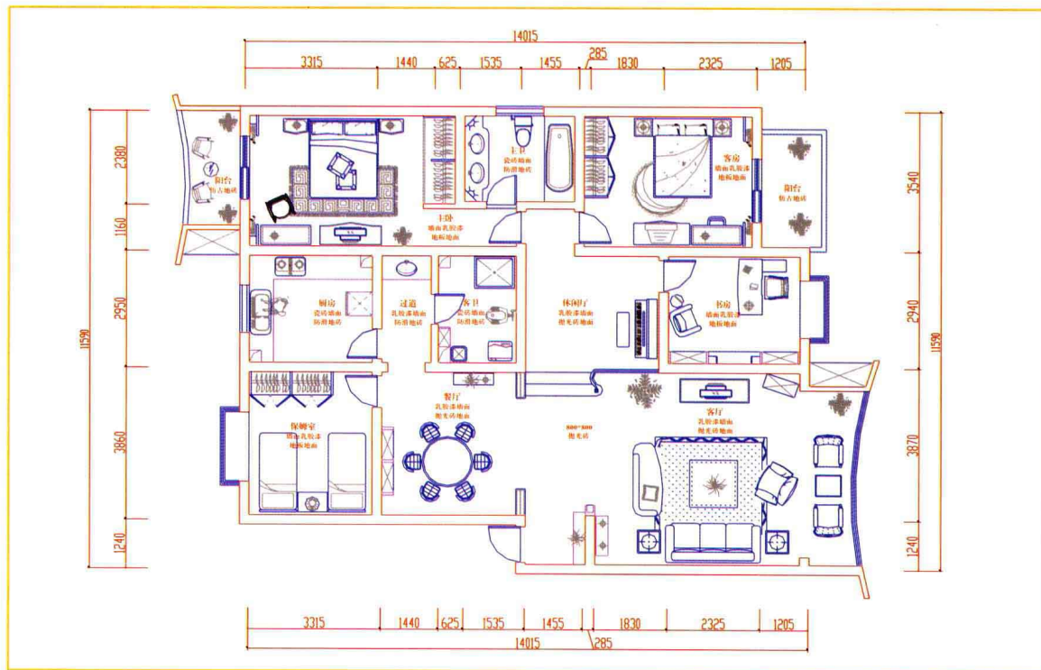
错层平面图
