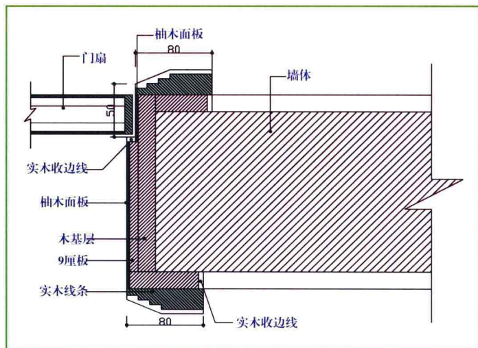
门套剖面图
