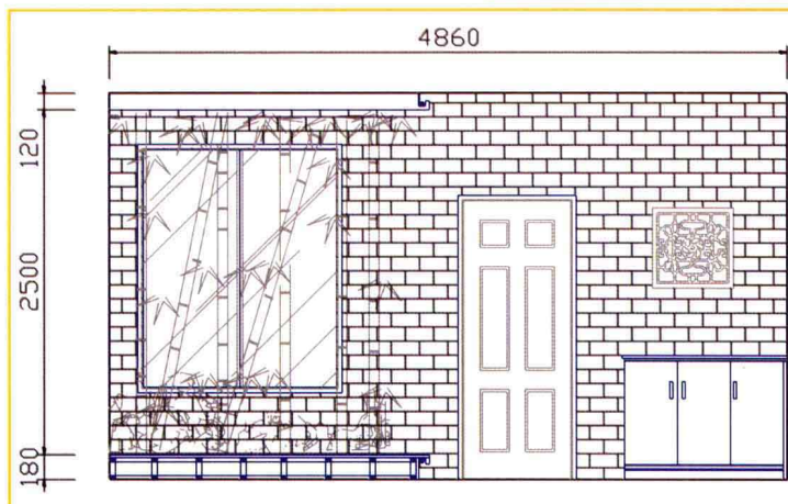
门厅装饰墙面
