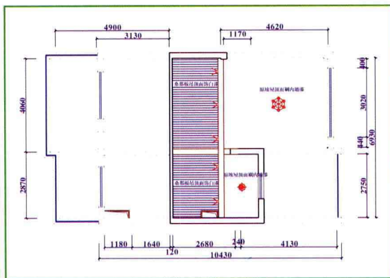
阁楼顶面图
