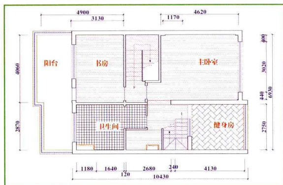
二层地面材质图
