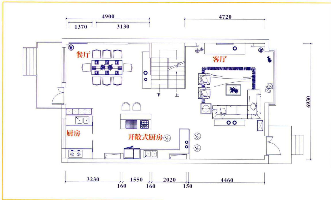
首层平面图
