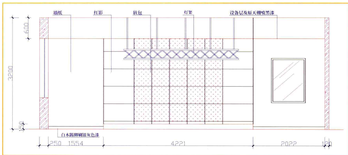
舞厅右立面图
