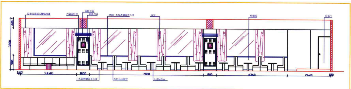
舞厅正立面图
