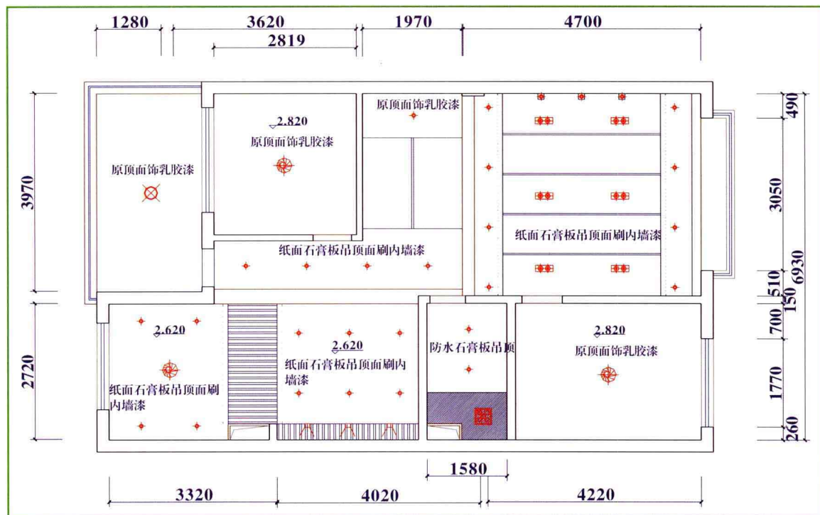
三层顶面图
