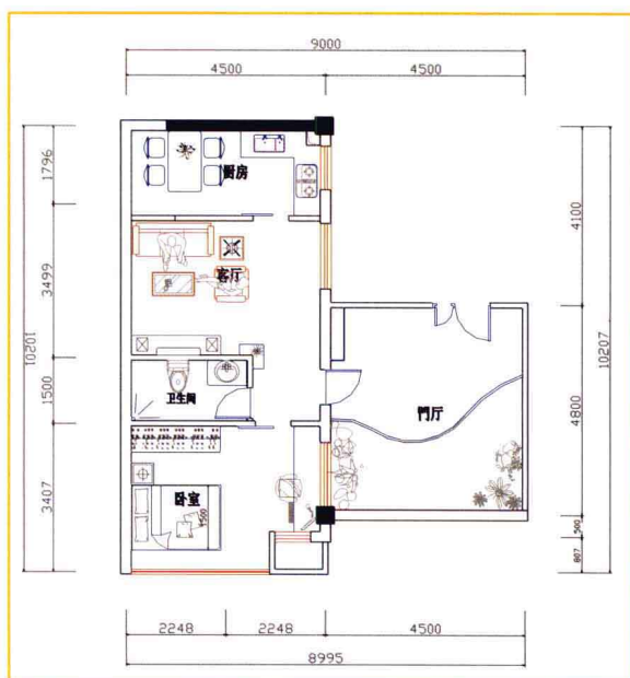
小户型平面图
