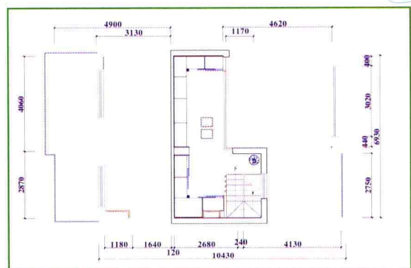
阁楼平面图
