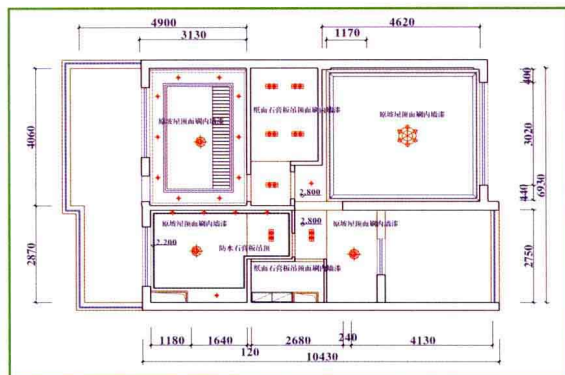
二层顶面图
