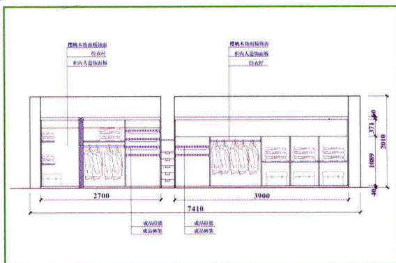
阁楼衣帽间立面图
