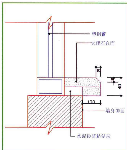
窗套剖面图
