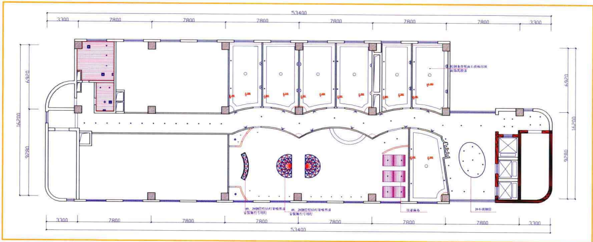
天棚图
