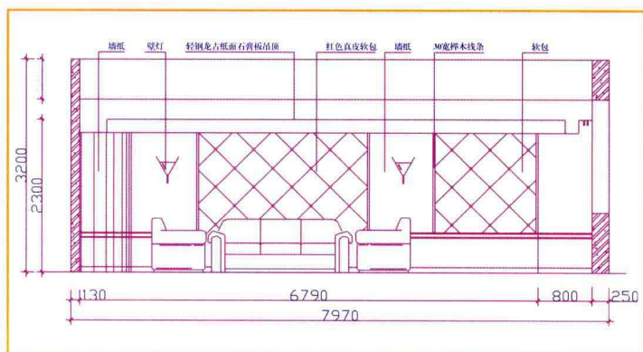
包间沙发背景立面图
