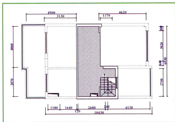
阁楼地面材质图
