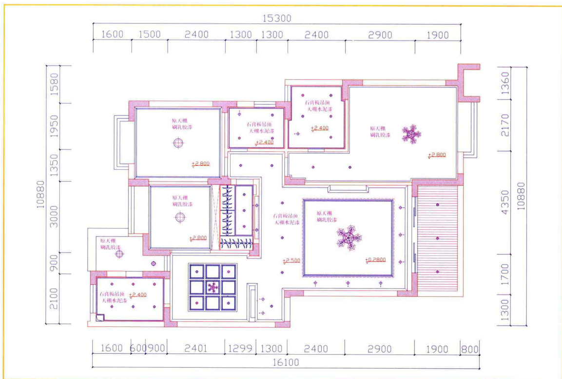
天棚图
