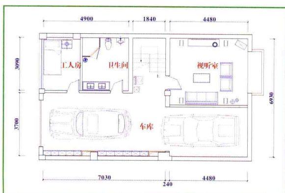
半地下室平面图
