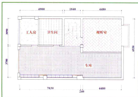
半地下室地面材质图
