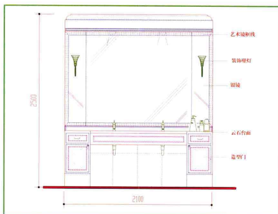
主卫立面
