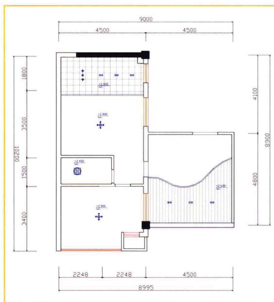
小户型顶面图
