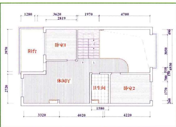
三层地面材质图
