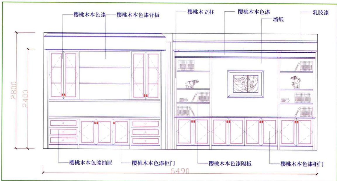
书柜立面图
