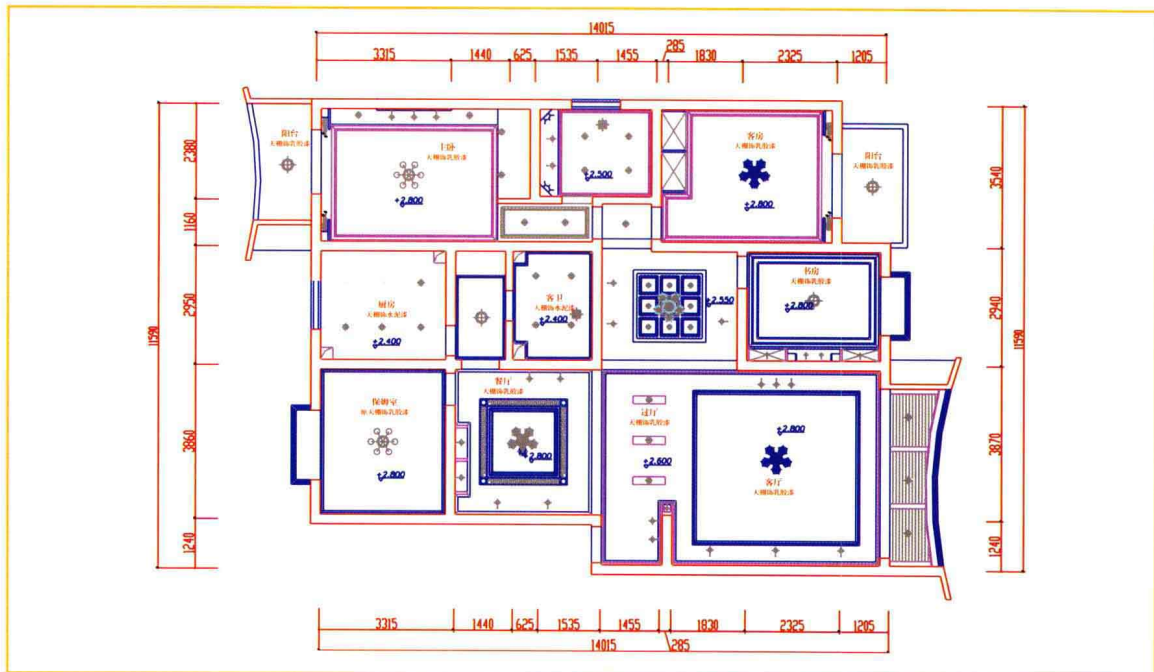
错层天棚图
