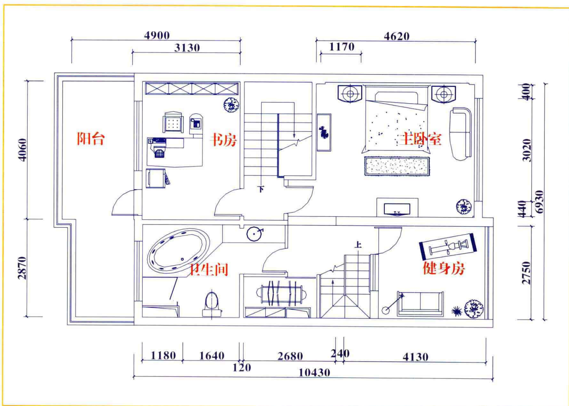
二层平面图
