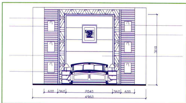
卧室立面图
