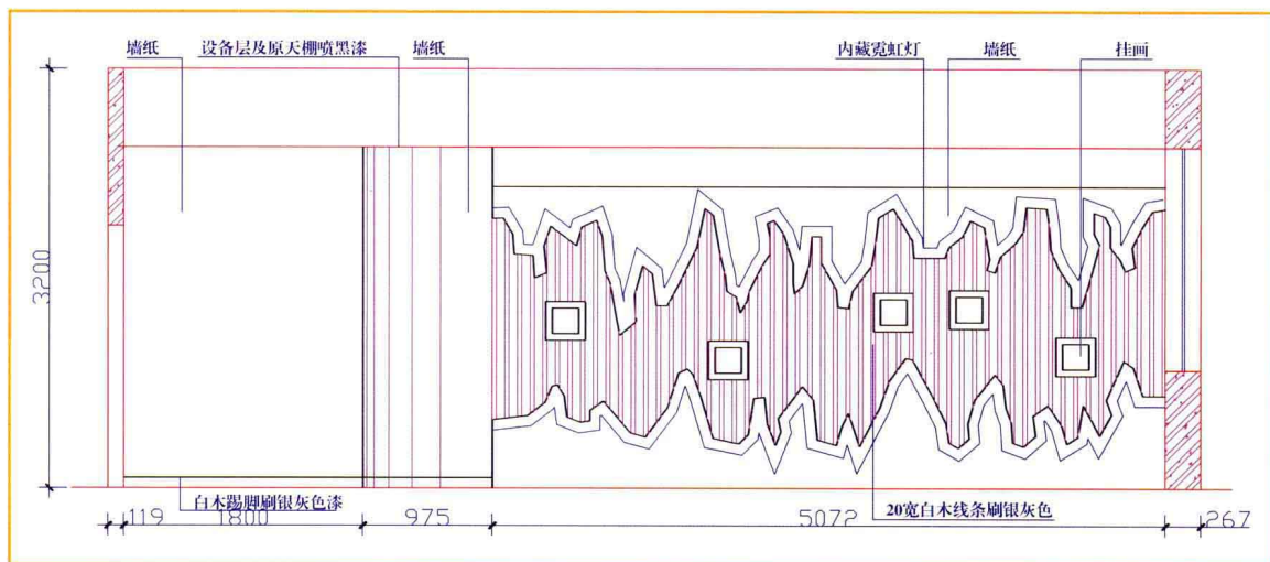
舞厅左立面图
