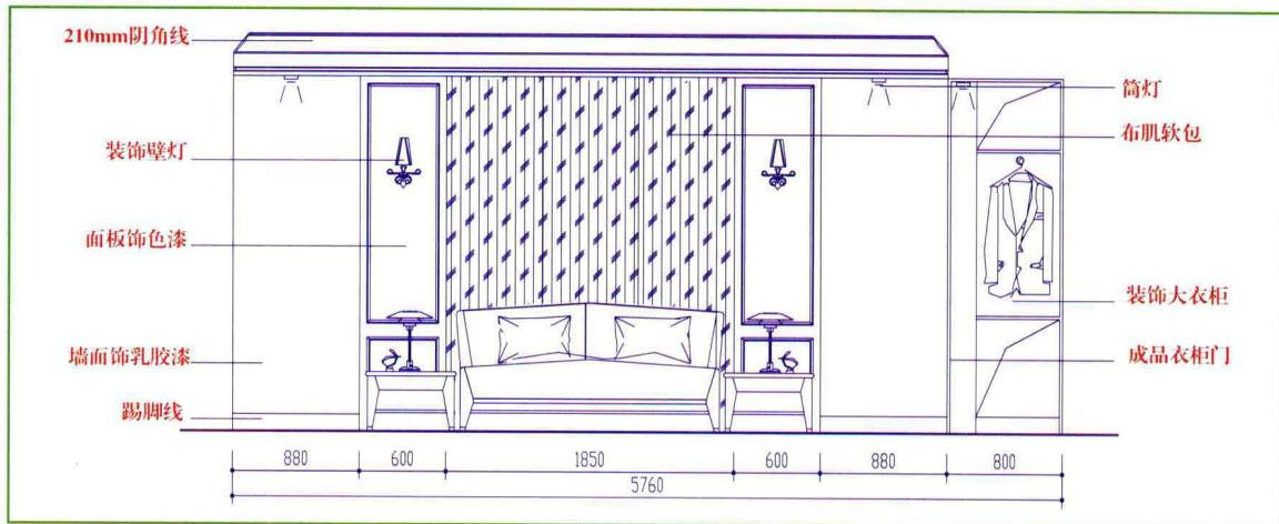
主卧床头背景立面图
