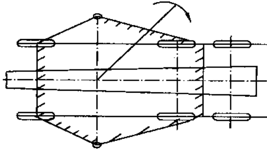
图 C.1 起重机前置 (双后桥)
