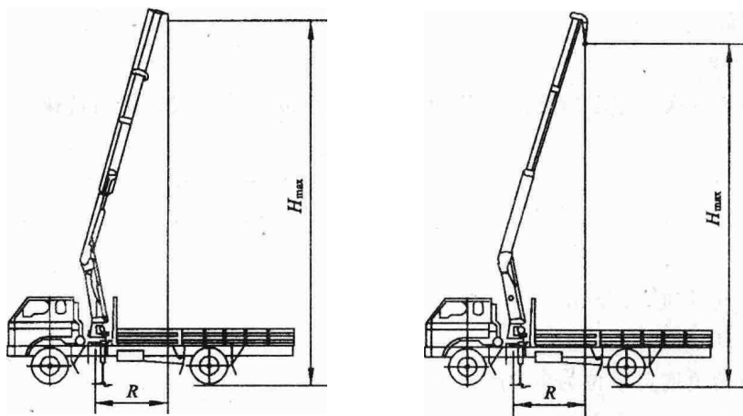
图 2 最大起升高度及其幅度的测量
