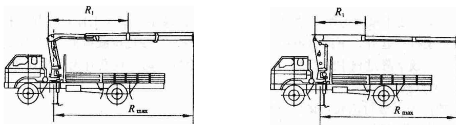
图 3 最大工作幅度及基本臂长度的测量
