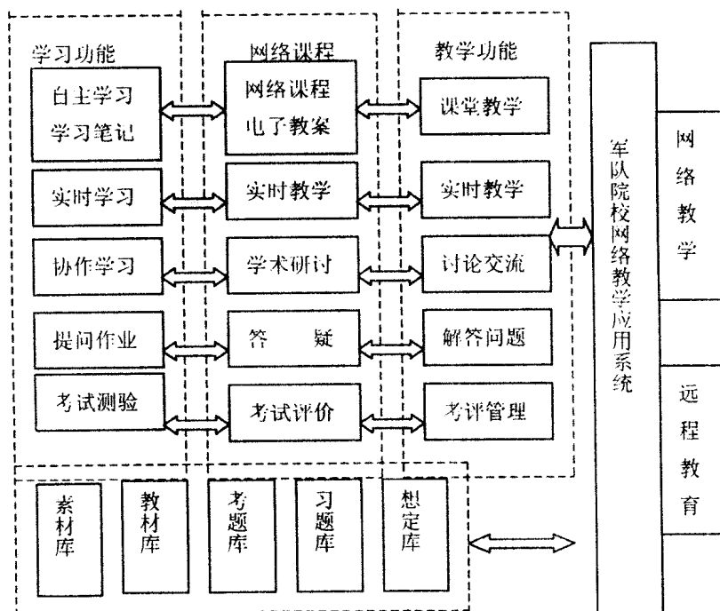
图7 军队院校教学信息资源的体系结构和功能示意图
