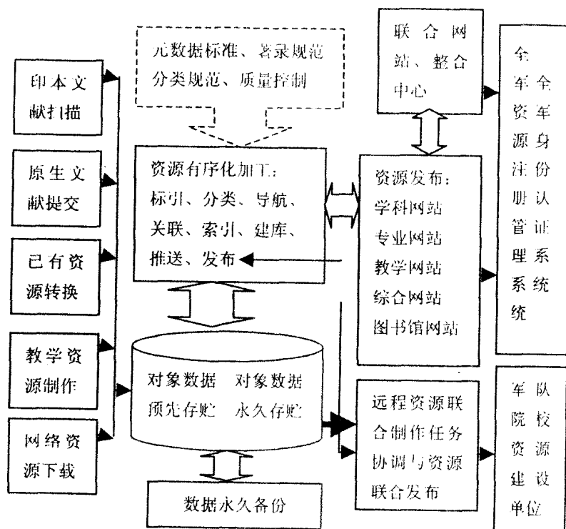
图 3 军队院校数字化信息资源技术应用系统的技术构成
