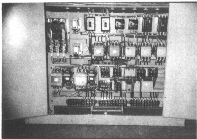
实 习 生 产 产 品 — 开 关 箱
