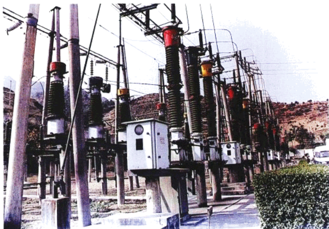
▲ 110千伏变电站变电区
