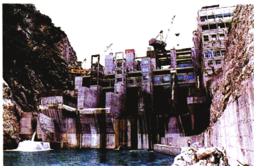
◀ 大河口电站坝前风貌
