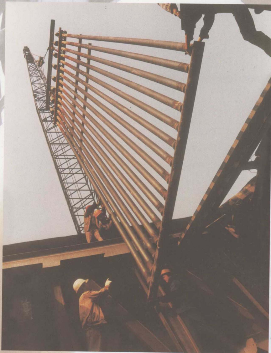
合成车间一段转化炉炉管 更换为新材料的薄壁管
