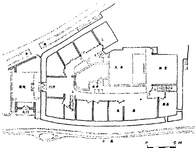
顺源楼底层平面图
