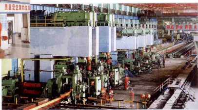
大连金牛股份公司初轧型材生产线
