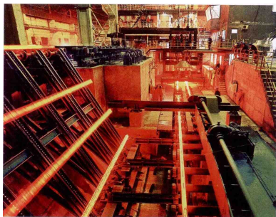
大连金牛股份公司第一炼钢厂连铸机
