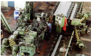
大连金牛股份公司银亮材厂盘条冷加工生产线
