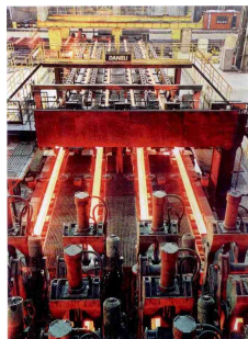
抚钢股份公司第一炼钢厂合金钢方坯连铸机
