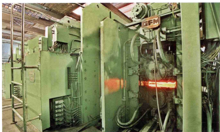
抚钢股份公司精轧厂WF-5-40型方扁钢精轧生产线
