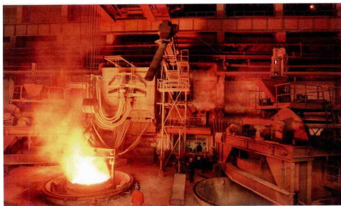
抚钢股份公司第二炼钢厂30/60吨 VOD/VHD炉外精炼炉
